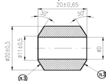
Кольцо уплотнительное СТП.07.005
